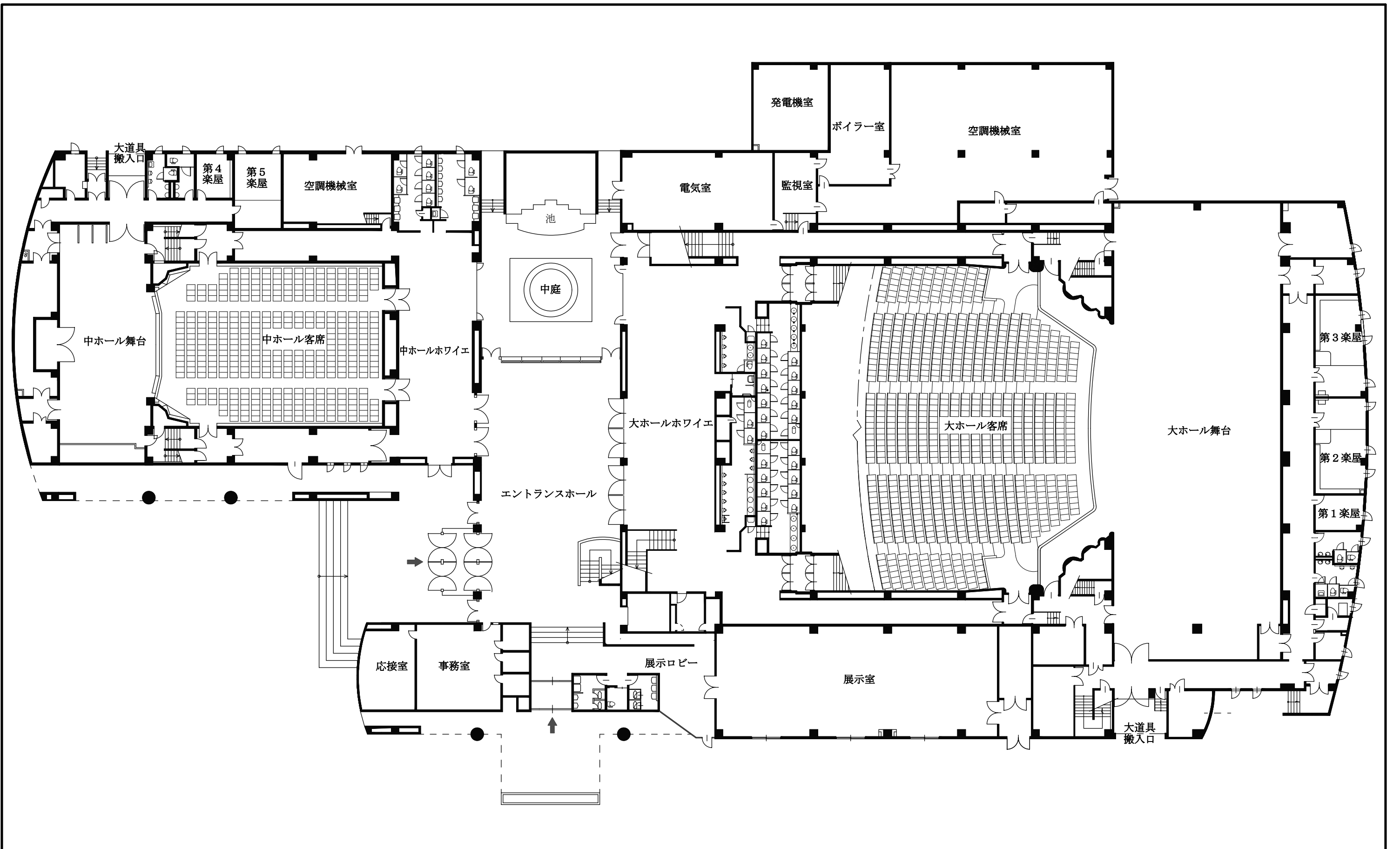
大館市民文化会館 1階平面図
